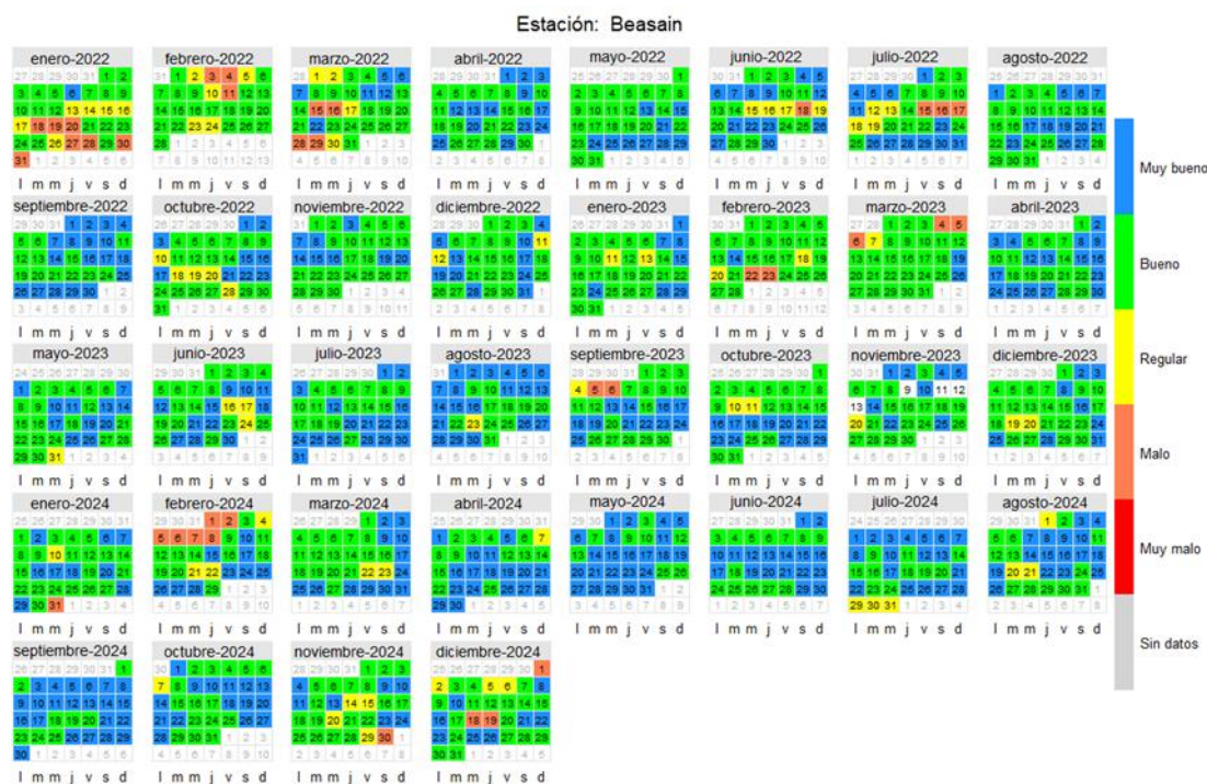
6. irudia: Eguneroko AKIa Beasaingo geltokiaren inguruan (2022-2024 aldia). Geuk egina. Datuak: EJ
